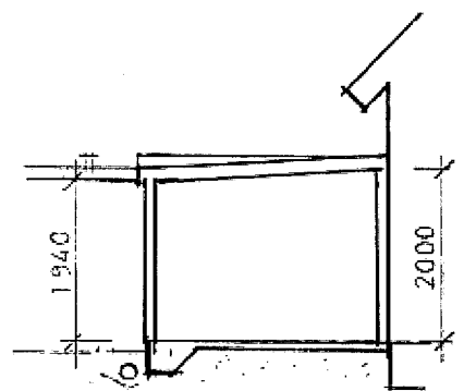
SEKTION A-A
