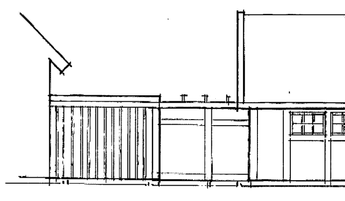
FASAD
