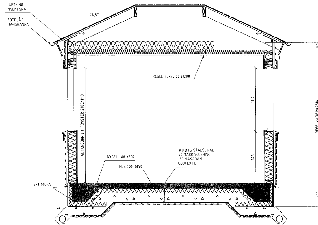
SEKTION B 1:20
