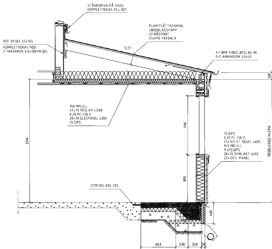
SEKTION A 1:20
