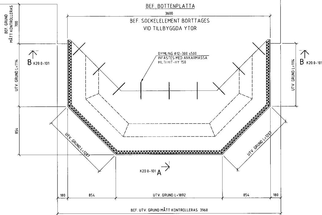
GRUNDPLAN -1:20-
